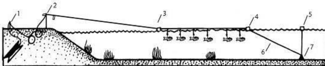
Рис. 5. Щучья резинка: 1 — колышек, надежно вбитый в берег; 2 — прут, в расщепе которого зажата основная леска; 3, 4 — поплавки; 5 — буй (иногда не применяется); 6 — резиновый амортизатор; 7 — груз.
