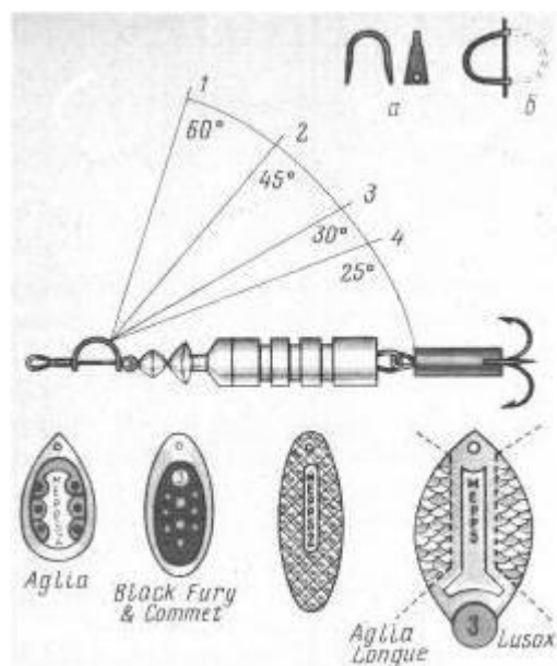
Рис. 25. Составные части вращающейся блесны и углы вращения различных по форме лепестков.
