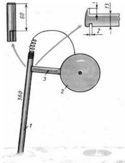
Рис. 18. Использование кружка в качестве элемента зимней жерлицы (конструкция В. Казанцева): 1 — стойка; 2 — кружок; 3 — рычаг.
