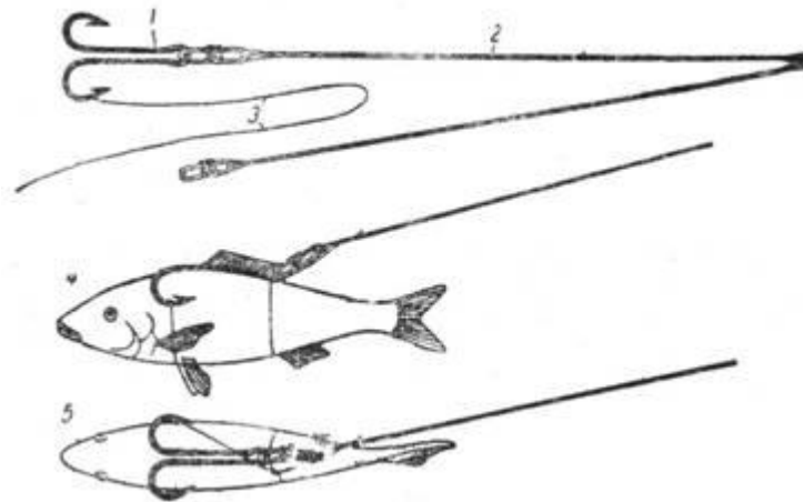
Рис. 10. Жерличная шлейка конструкции И. Михайлова: 1 — двойник; 2 — двухколенный поводок; тонкая гибкая проволока для шлейки; 4 и 5 — впрыженная рыбка.
