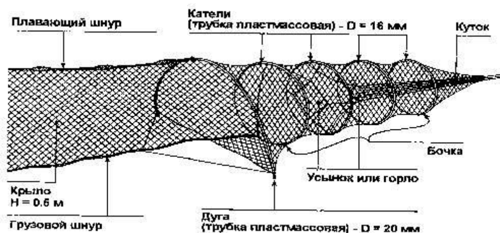
Рис. 49. Устройство современной мережи (для удобства изображено лишь одно крыло).
