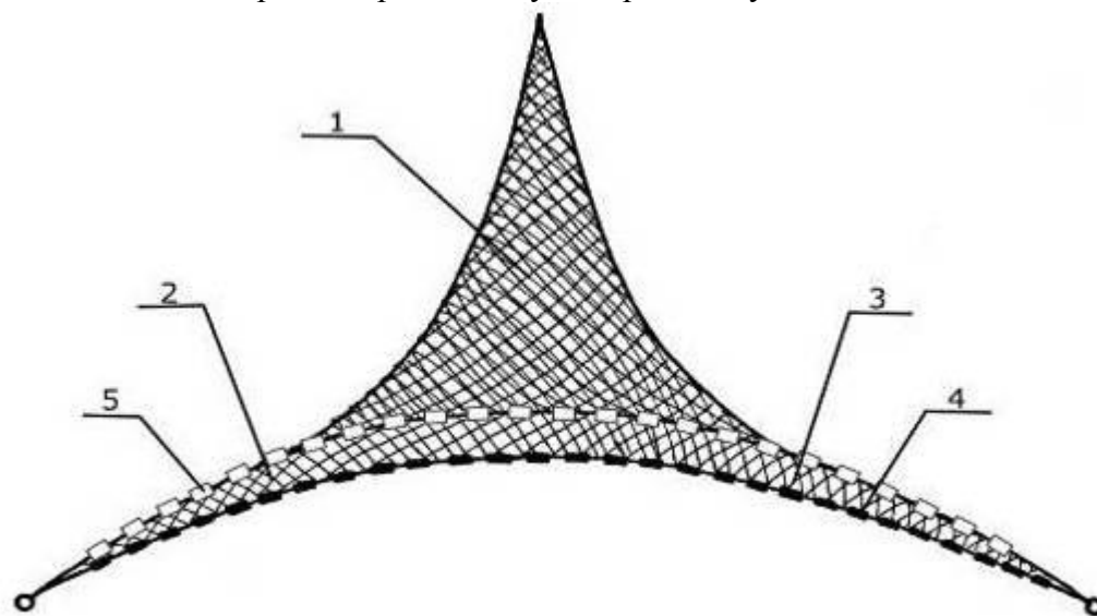
Рис. 39. Короткий бредень для речной ловли (вид сверху): 1 — мотня; 2, 3 — крылья; 4 — грузовой шнур; 5 — наплавной шнур.
