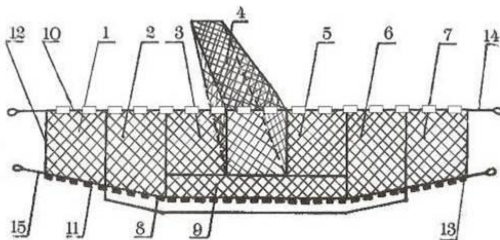
Рис. 38. Бредень и его составные части: 1 — правое крыло (2 часть); 2 — правое крыло (1 часть), 3 — правый привод; 4 — мотня; 5 — левый привод; 6 — левое крыло (2 часть); 7 — левое крыло (1 часть); 8 — подзор; 9 — сорочка; 10 — верхняя подбора; 12 — правый кляч; 13 — левый кляч; 14 — верхняя чалка; 15 — нижняя чалка.
