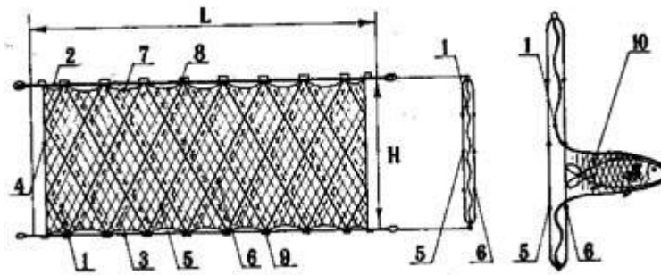
Рис 37. Трехстенная сеть (путанка) и принцип ее действия: 1 — сетное полотно; 2 — верхняя подбора; 3 — нижняя подбора; 4 — боковая подбора (пожилина); 5, 6 — режа, 7 — посадочная нитка; 8 — поплавок; 9 — грузило; 10 — сетной мешок (карман).
