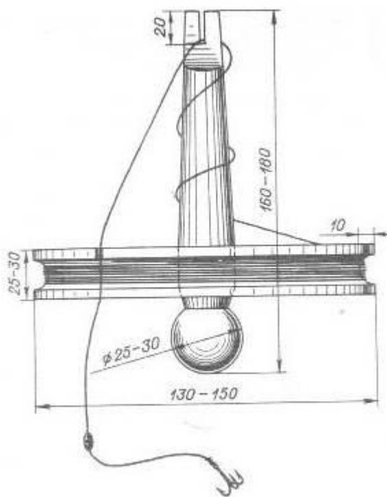
Рис. 11. Кружок в сборе
