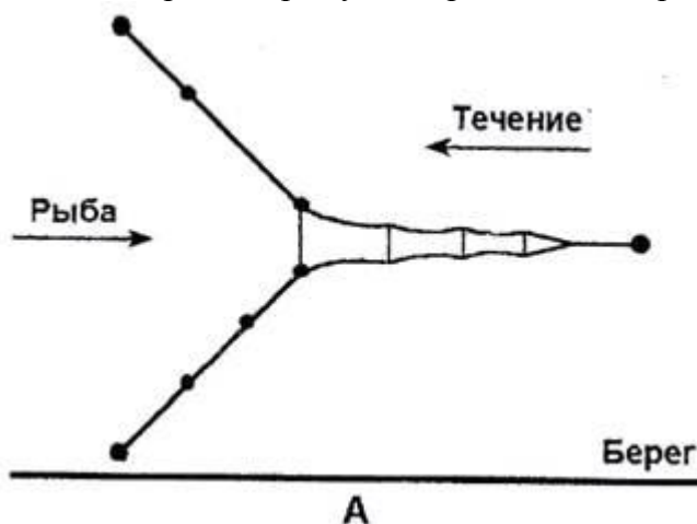
Рис. 50. Положение двухкрыльной мережи при ходе рыбы в верховья реки. При обратном скатывании снасть разворачивается на 180 градусов.
